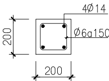
MC 7A-7A
