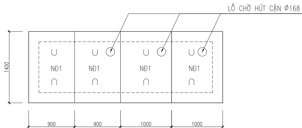
MẶT BẰNG NẮP ĐÀN
