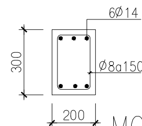
MÔNG M-3
