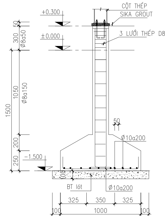
MẶT CẮT 2-2
