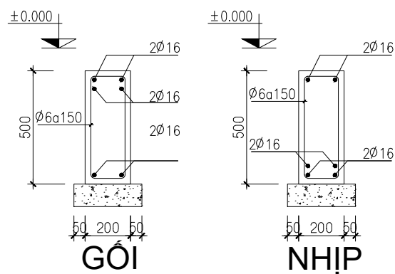
ĐÀ KIỀNG ĐK-1 TL 1/25
