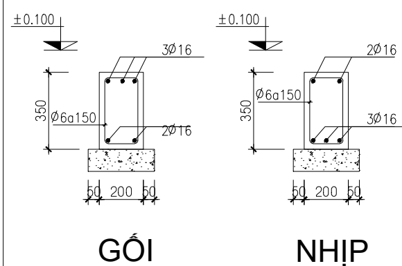
ĐÀ KIỀNG ĐK-3 TL 1/25
