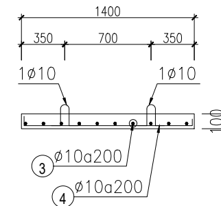
MẶT CẮT 1-1
