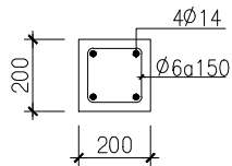
MC 6A-6A TL 1/25
