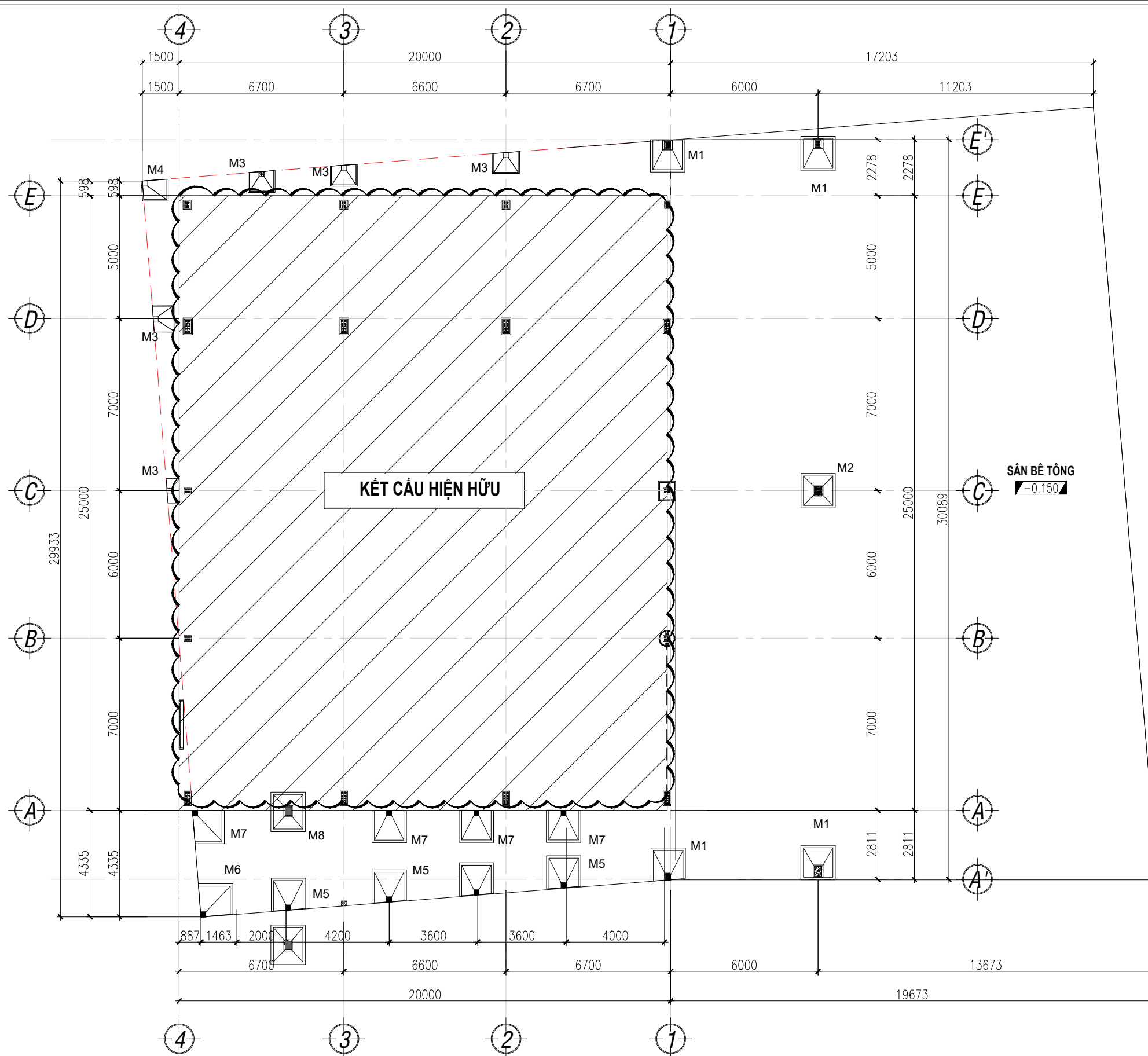
MẶT BẰNG MÓNG NÂNG CẤP TL: 1/100
