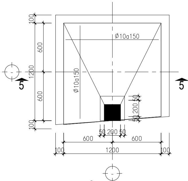
MÓNG M-5 TL 1/25
