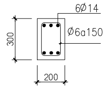
MC 4A-4A TL 1/25
