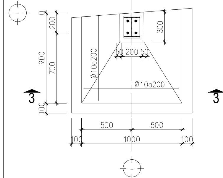
MÔNG M-3
