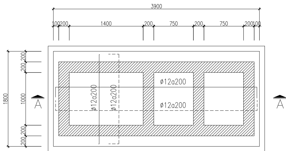
MẶT BẰNG BỐ TRÍ THÉP BẢN ĐÁY
