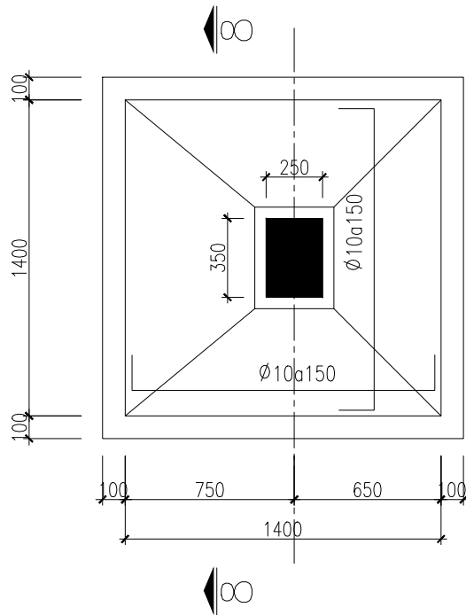
CHI TIẾT MÓNG M8
