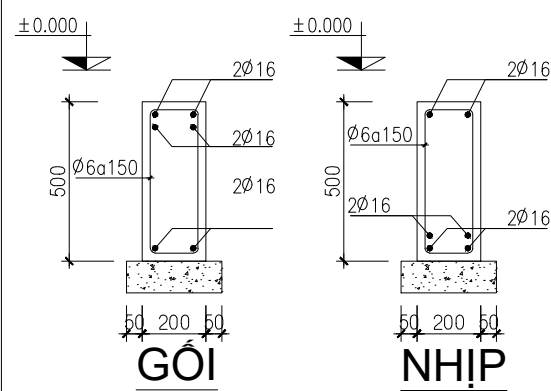
ĐÀ KIỀNG ĐK-2 TL 1/25
