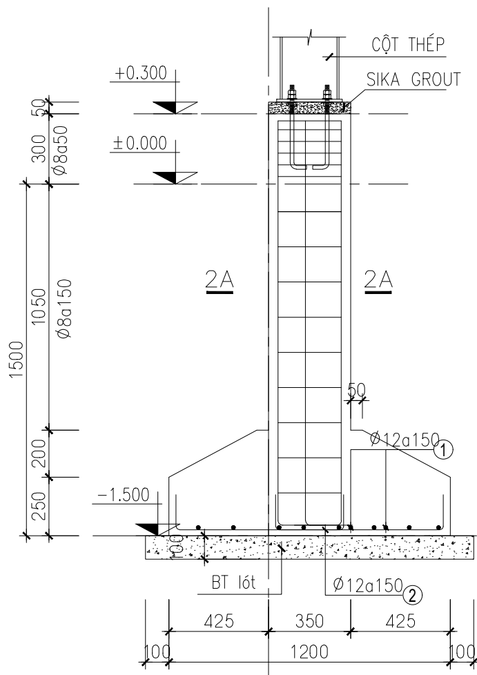
MC 2A-2A
