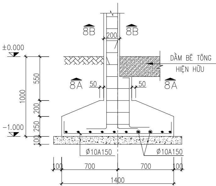
MẶT CẮT 8-8
