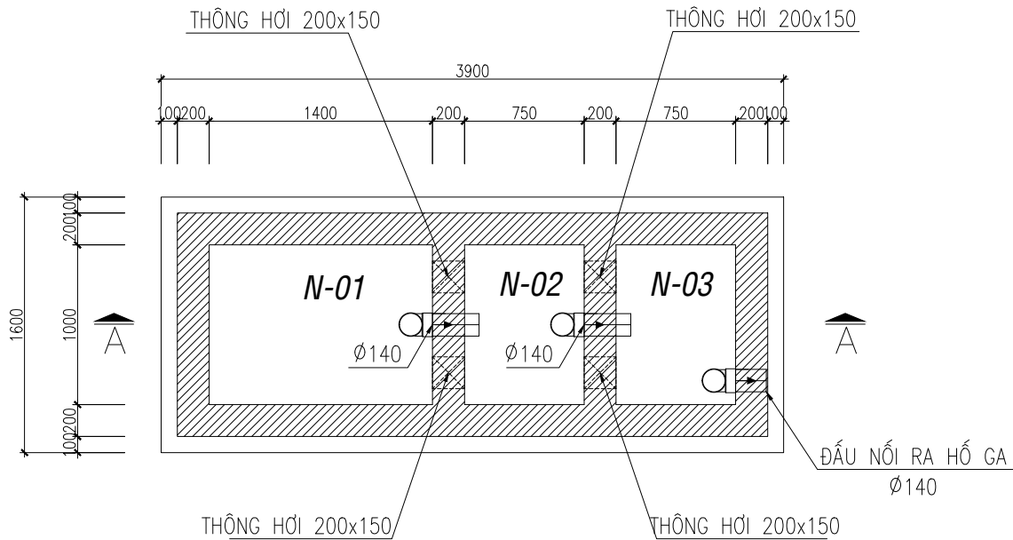
MẶT BẰNG BỂ TỰ HOẠI
