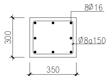
MC 1A-1A
