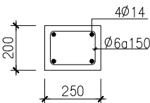
MẶT CẮT 8B-8B
