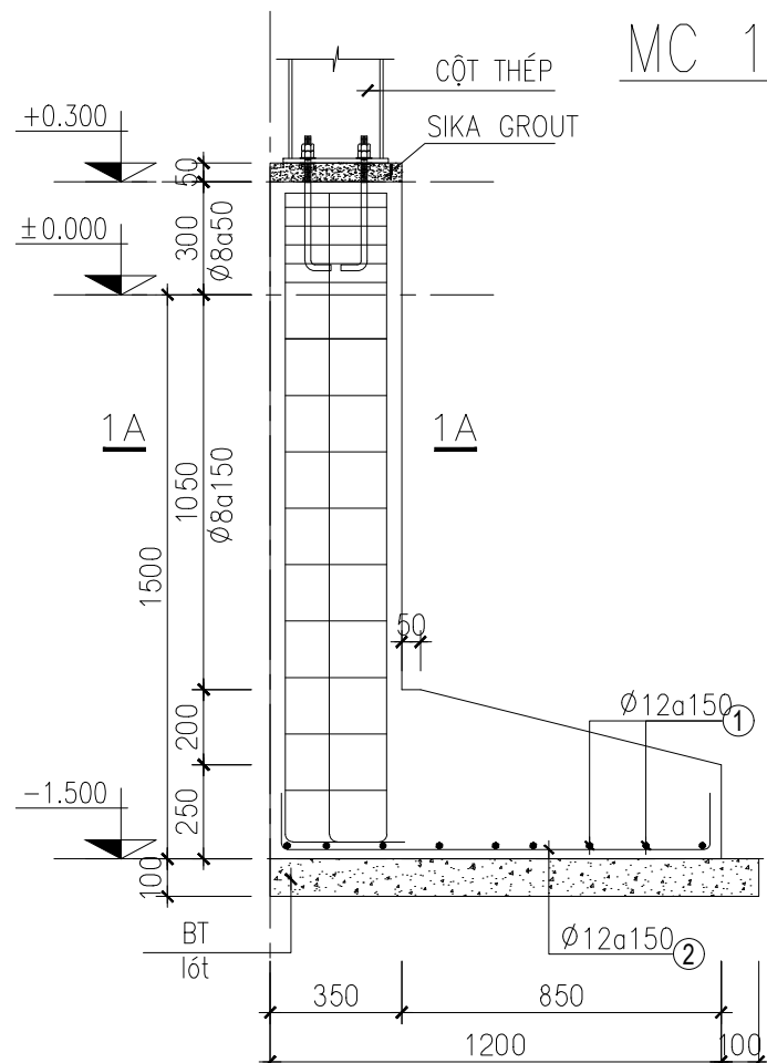
MẶT CẮT 1-1
