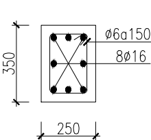
MẶT CẮT 8A-8A
