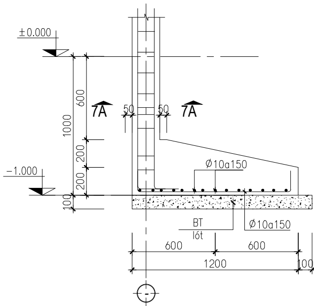
MẶT CẮT 7-7
