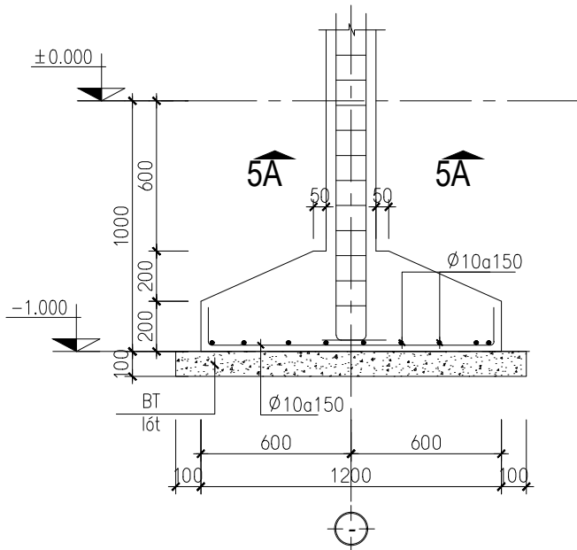
MẶT CẮT 5-5 TL 1/25
