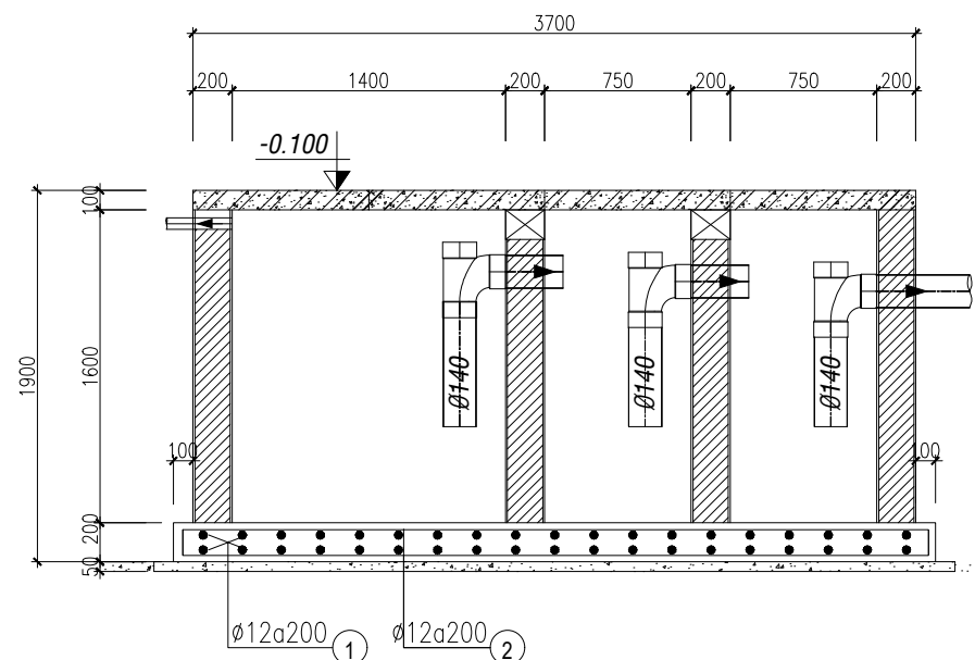
MẶT CẮT A-A BỐ TRÍ THÉP
