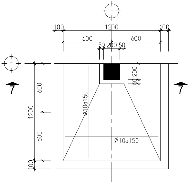
MÓNG M-7
